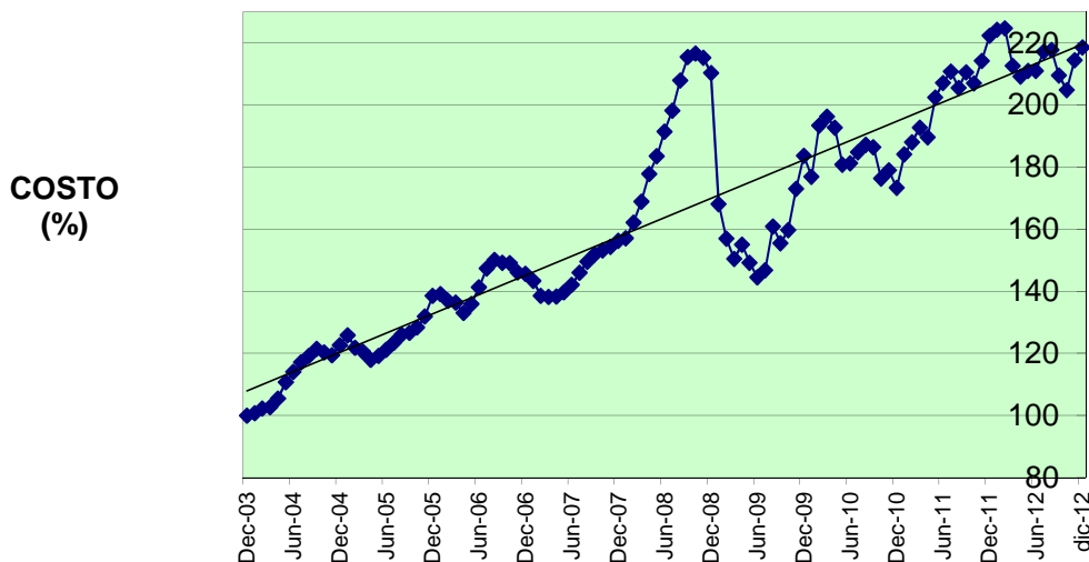
COSTO DEL kWh - TARIFA OM - Región Sur 2004-2012 100 = $0.618 EN DIC 2003
