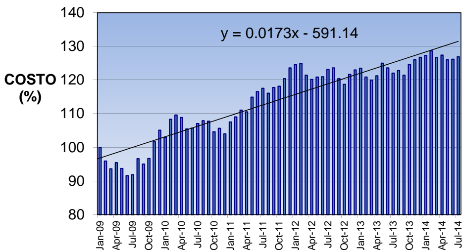
COSTO DEL kWh - TARIFA HT PUNTA - Región Sur 2009 - 2013 100 = $1.8769 EN ENERO 2009
