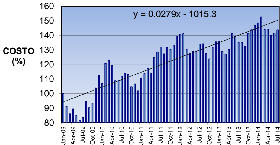
COSTO DEL kWh - TARIFA HT INTERMEDIA - Región Sur 2009 - 2013 100 = $0.7824 EN ENERO 2009
